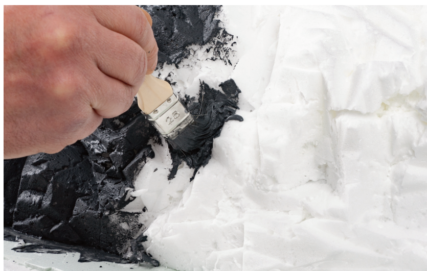
Einpinseln mit Geländebau-Spachtelmasse Art. 170654, um die verbleibenden Poren zu schließen.
