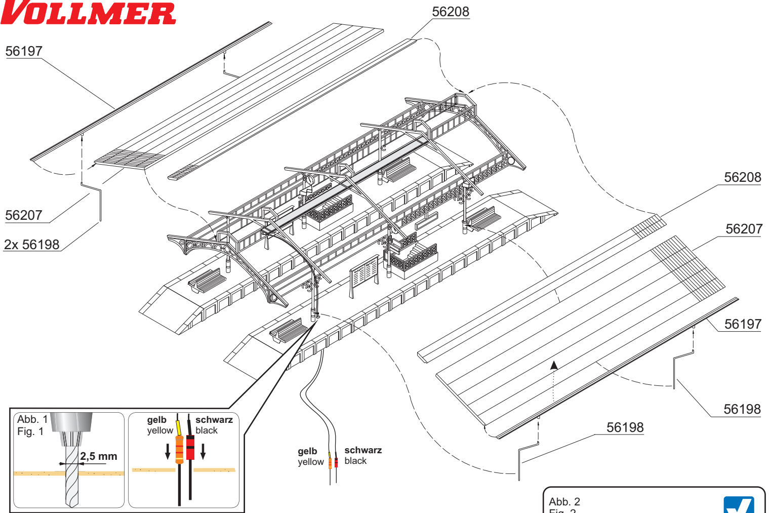
Am Einbauort ein Loch (Ø 2,5 mm) zur Montage bohren (Abb. 1). Drill a hole (Ø 2,5 mm) at the mounting place (fig. 1).
