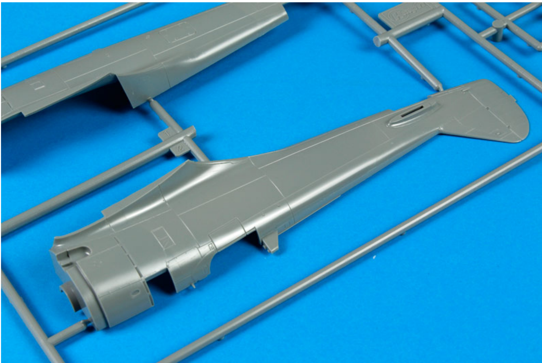
Detailaufnahmen der Spritzgussteile
